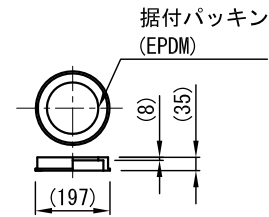
標準付属品 外形図 S=1/20
